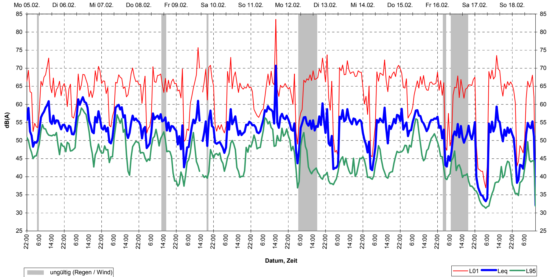
Schalldruckpegel (Stundenmittel) Denkendorf, MP4 05.02.01 bis 19.02.01
