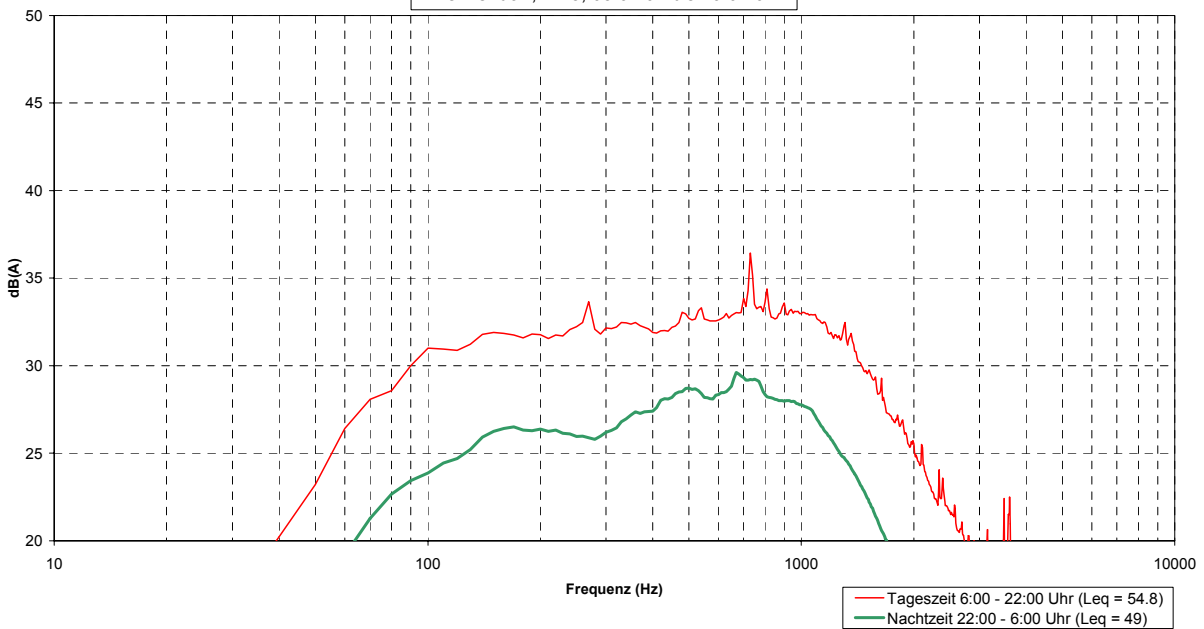
gemittelte Spektren aller gültigen Messungen Denkendorf, MP5, 05.02.01 bis 19.02.01
