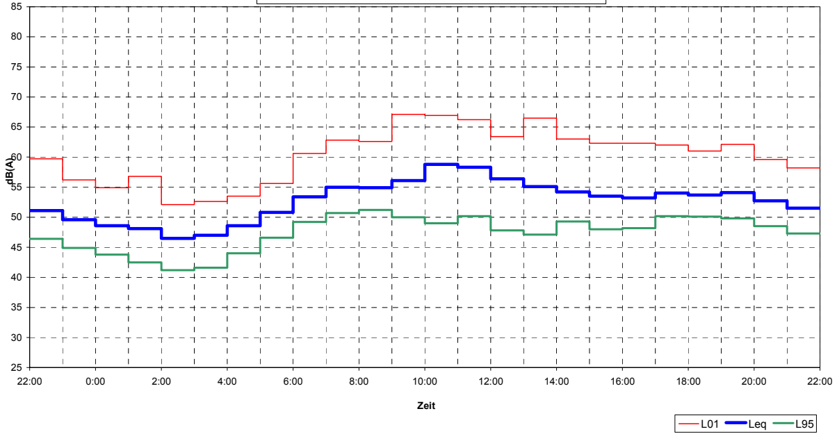
Tagesgang der gemittelten Pegel aller gültigen Messungen Denkendorf, MP5, 05.02.01 bis 19.02.01
