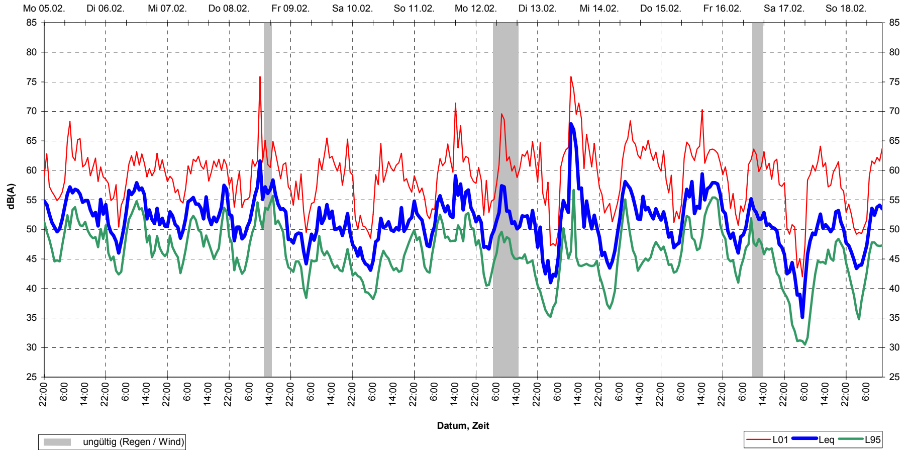
Schalldruckpegel (Stundenmittel) Denkendorf, MP5 05.02.01 bis 19.02.01
