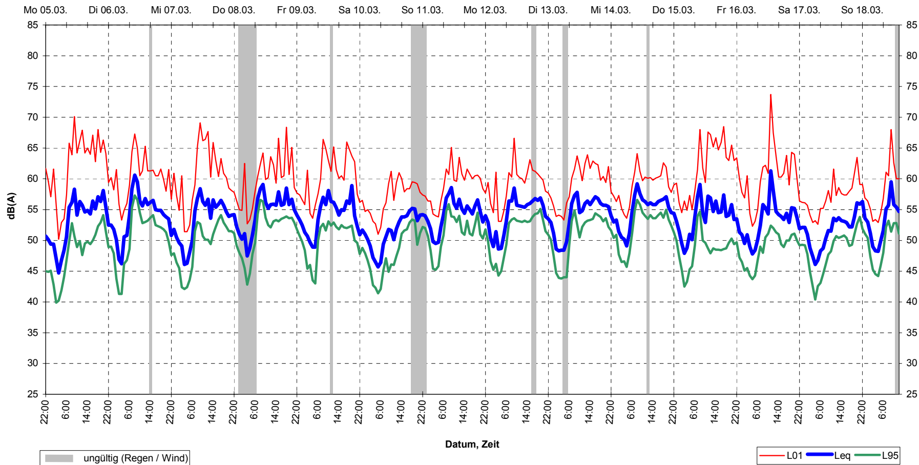
Schalldruckpegel (Stundenmittel) Denkendorf, MP10 05.03.01 bis 19.03.01
