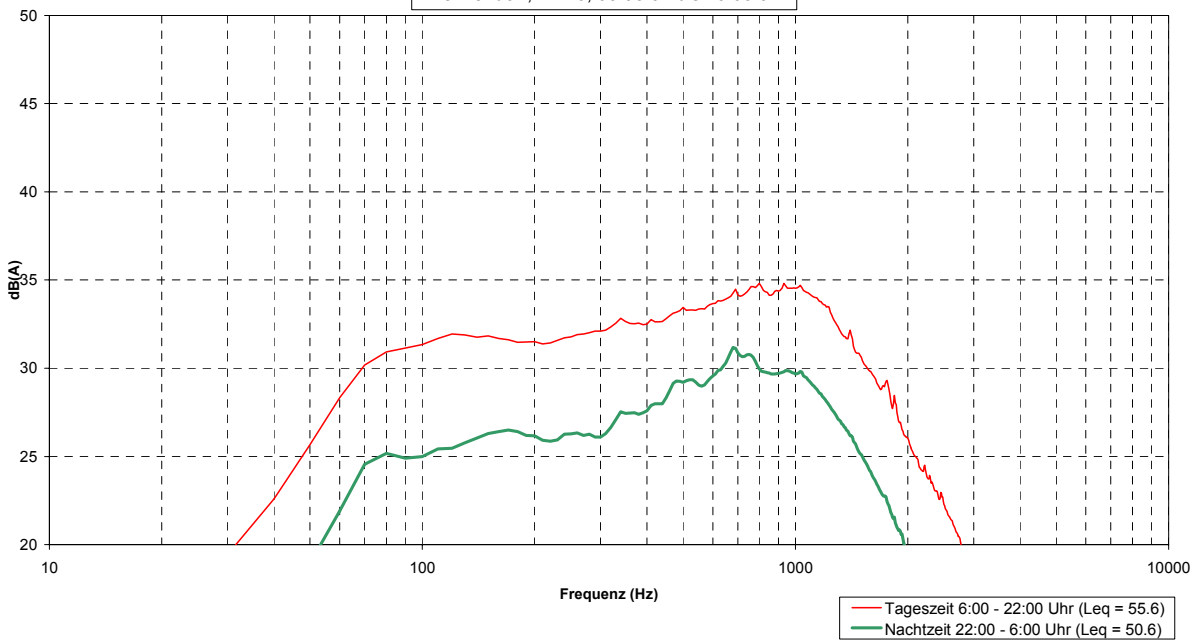
gemittelte Spektren aller gültigen Messungen Denkendorf, MP10, 05.03.01 bis 19.03.01
