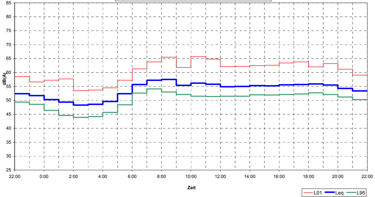
Tagesgang der gemittelten Pegel aller gültigen Messungen Denkendorf, MP10, 05.03.01 bis 19.03.01
