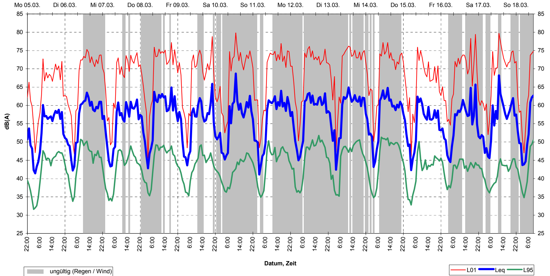
Schalldruckpegel (Stundenmittel) Filderstadt, MP11 05.03.01 bis 19.03.01
