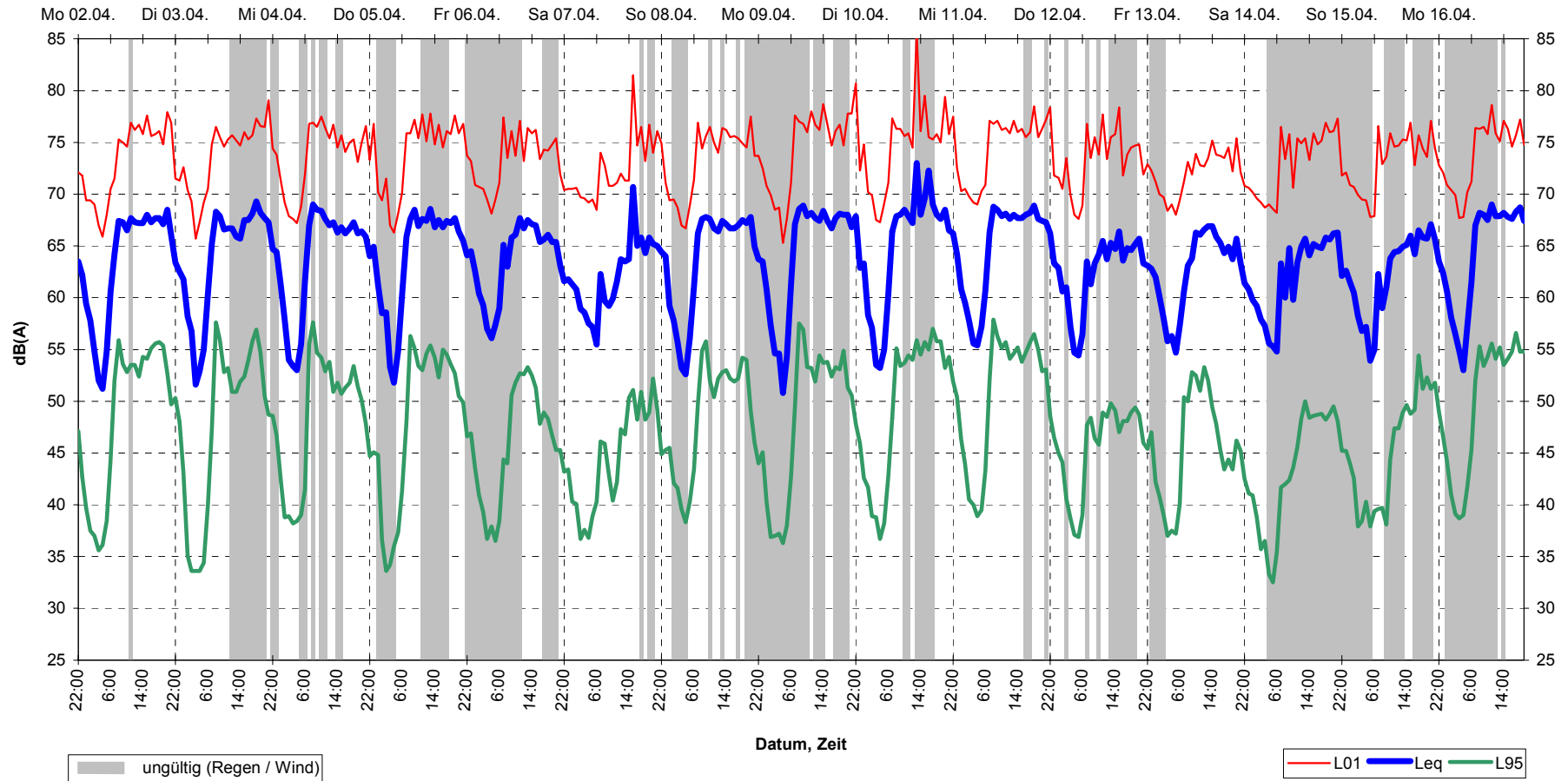
Schalldruckpegel (Stundenmittel) Filderstadt, MP17 02.04.01 bis 17.04.01
