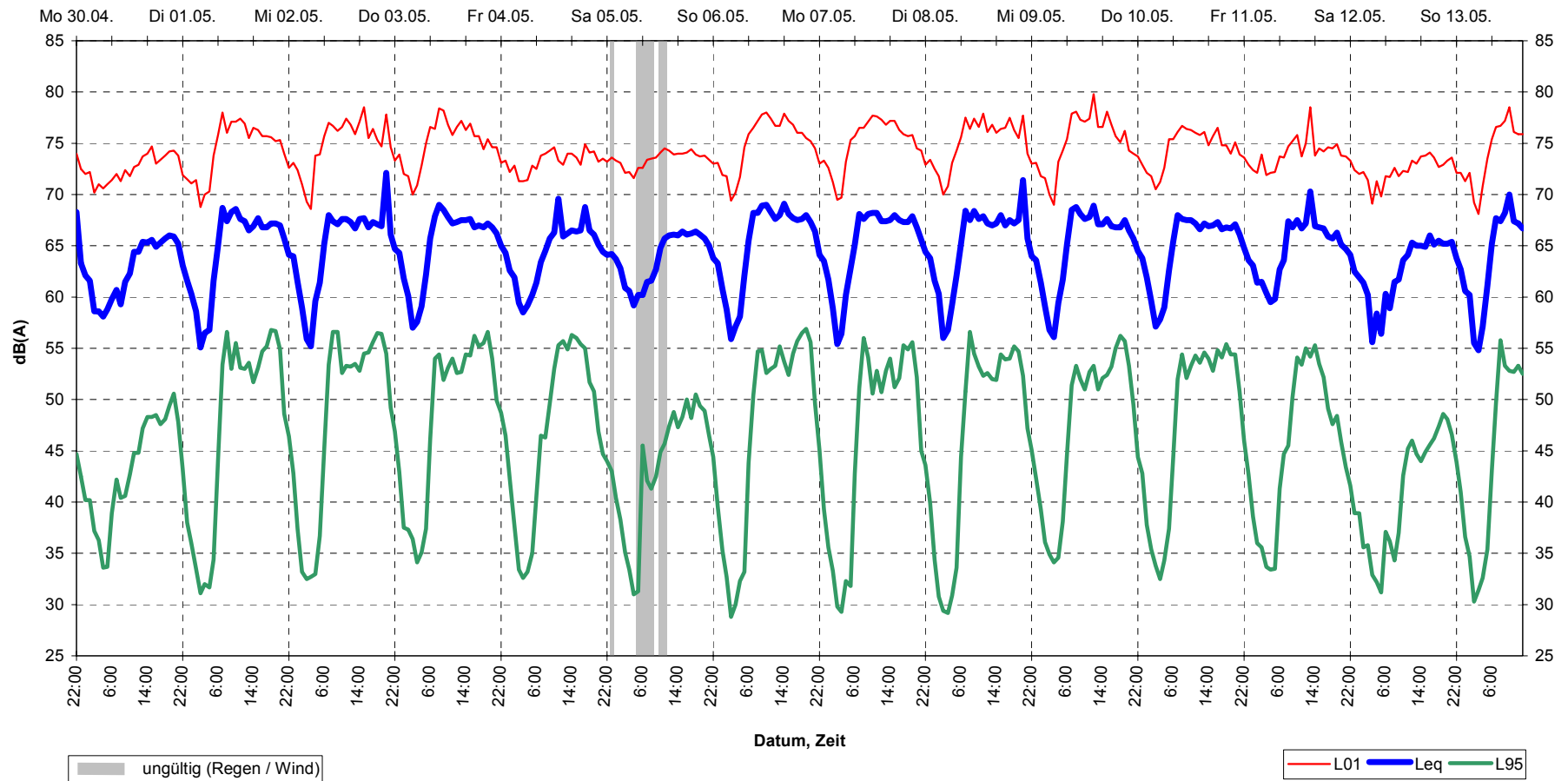
Schalldruckpegel (Stundenmittel) Filderstadt, MP20 30.04.01 bis 14.05.01
