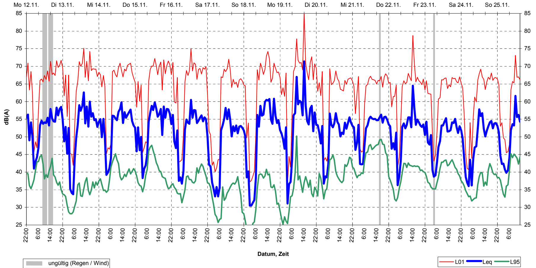
Schalldruckpegel (Stundenmittel) Ostfildern, MP22 12.11.01 bis 26.11.01
