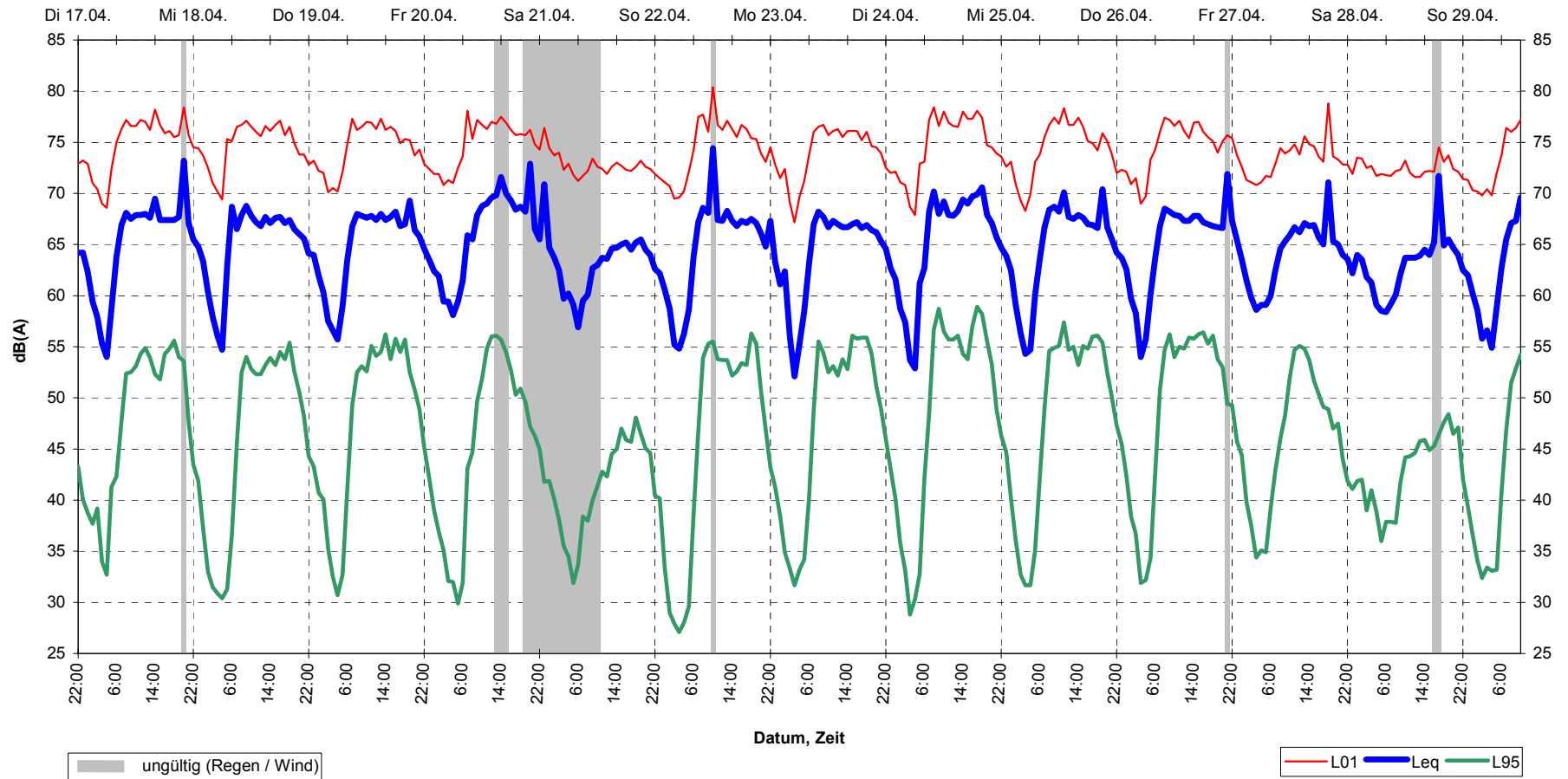
Schalldruckpegel (Stundenmittel) Filderstadt, MP23 17.04.01 bis 30.04.01
