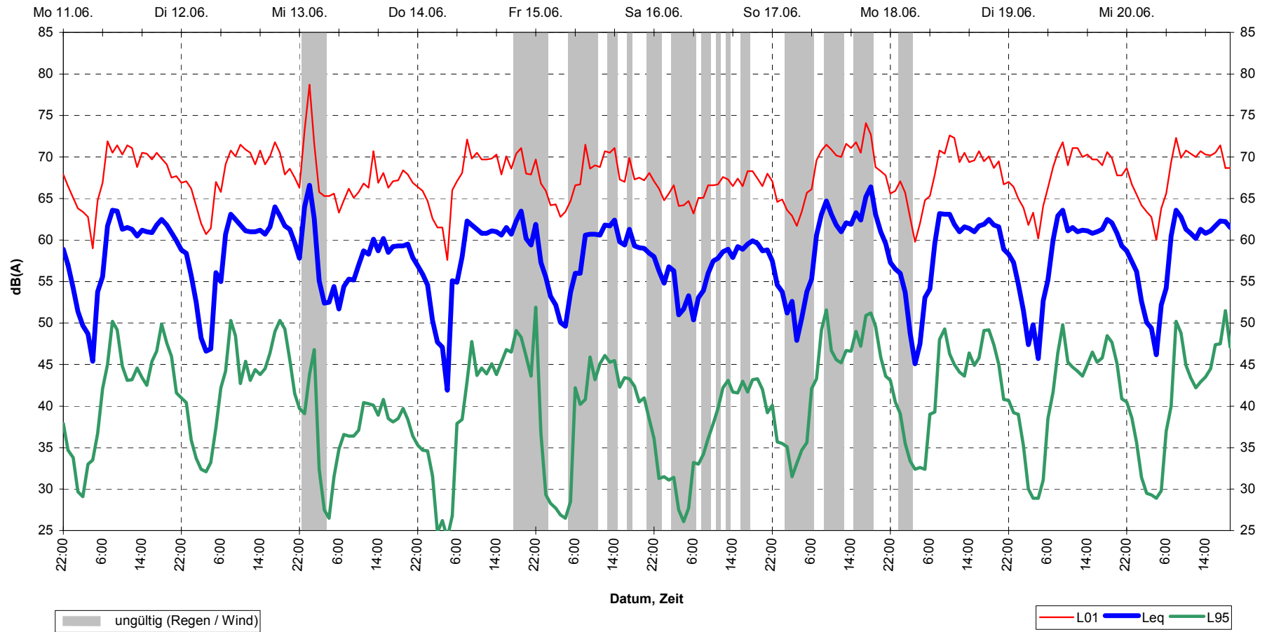
Schalldruckpegel (Stundenmittel) Leinf.-Echterd., MP31 11.06.01 bis 21.06.01
