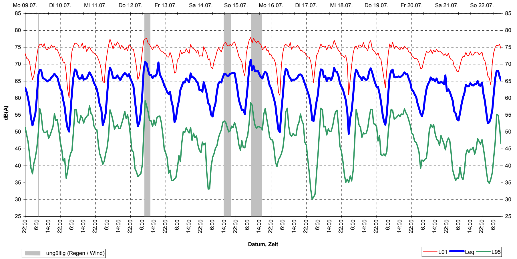
Schalldruckpegel (Stundenmittel) Leinf.-Echterd., MP37 09.07.01 bis 23.07.01
