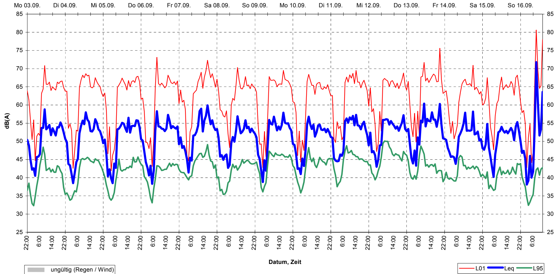
Schalldruckpegel (Stundenmittel) Stuttgart, MP42 03.09.01 bis 17.09.01
