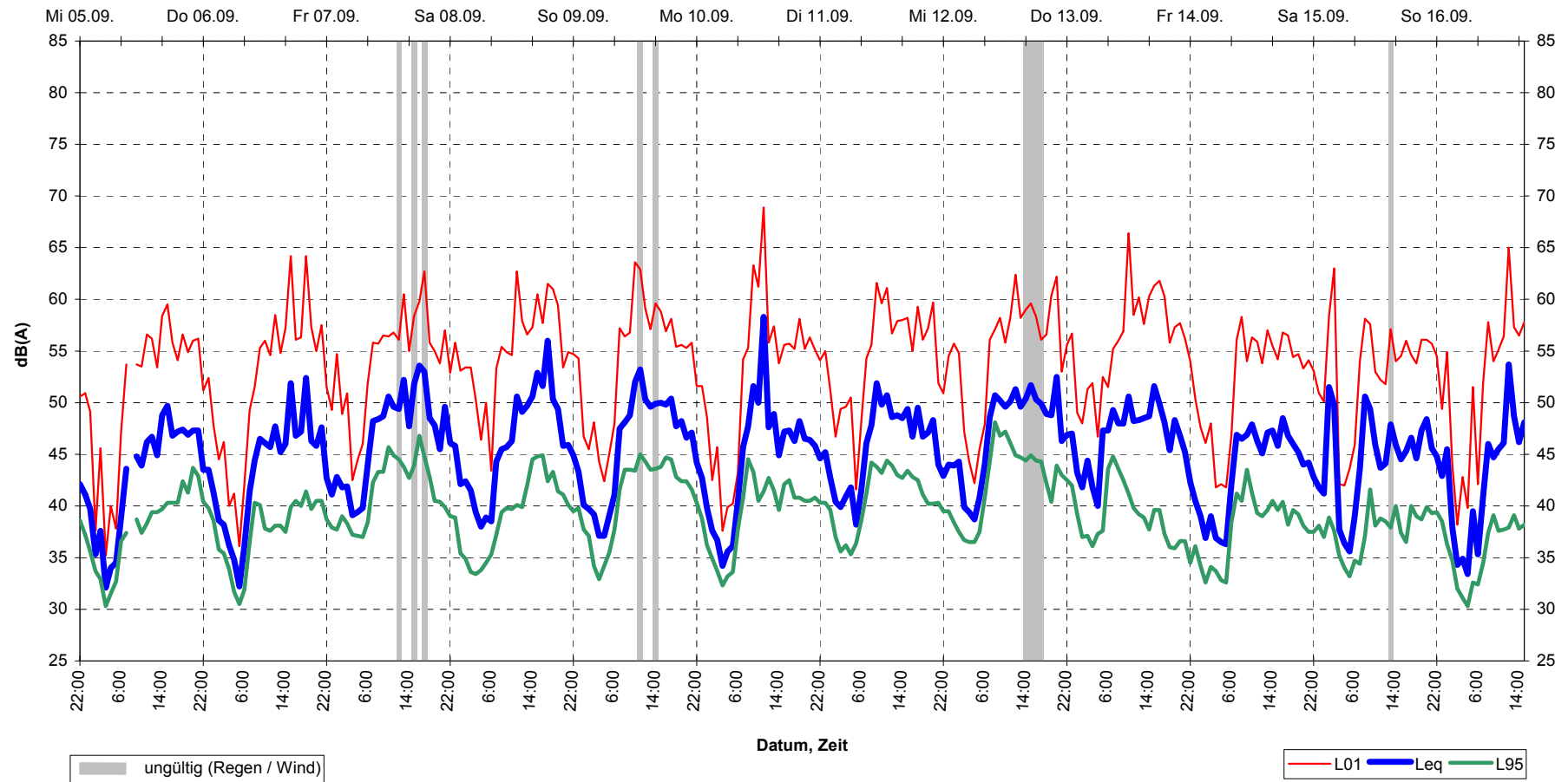
Schalldruckpegel (Stundenmittel) Stuttgart, MP45 05.09.01 bis 17.09.01
