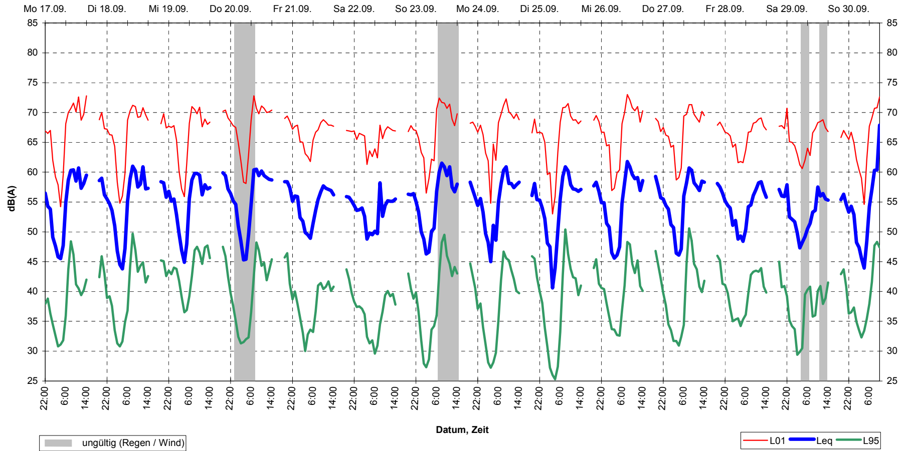
Schalldruckpegel (Stundenmittel) Stuttgart, MP48 17.09.01 bis 01.10.01
