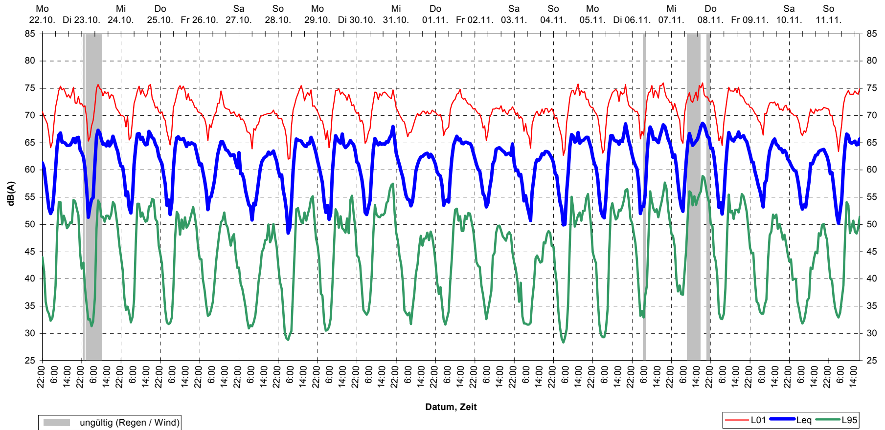
Schalldruckpegel (Stundenmittel) Ostfildern, MP56 22.10.01 bis 12.11.01
