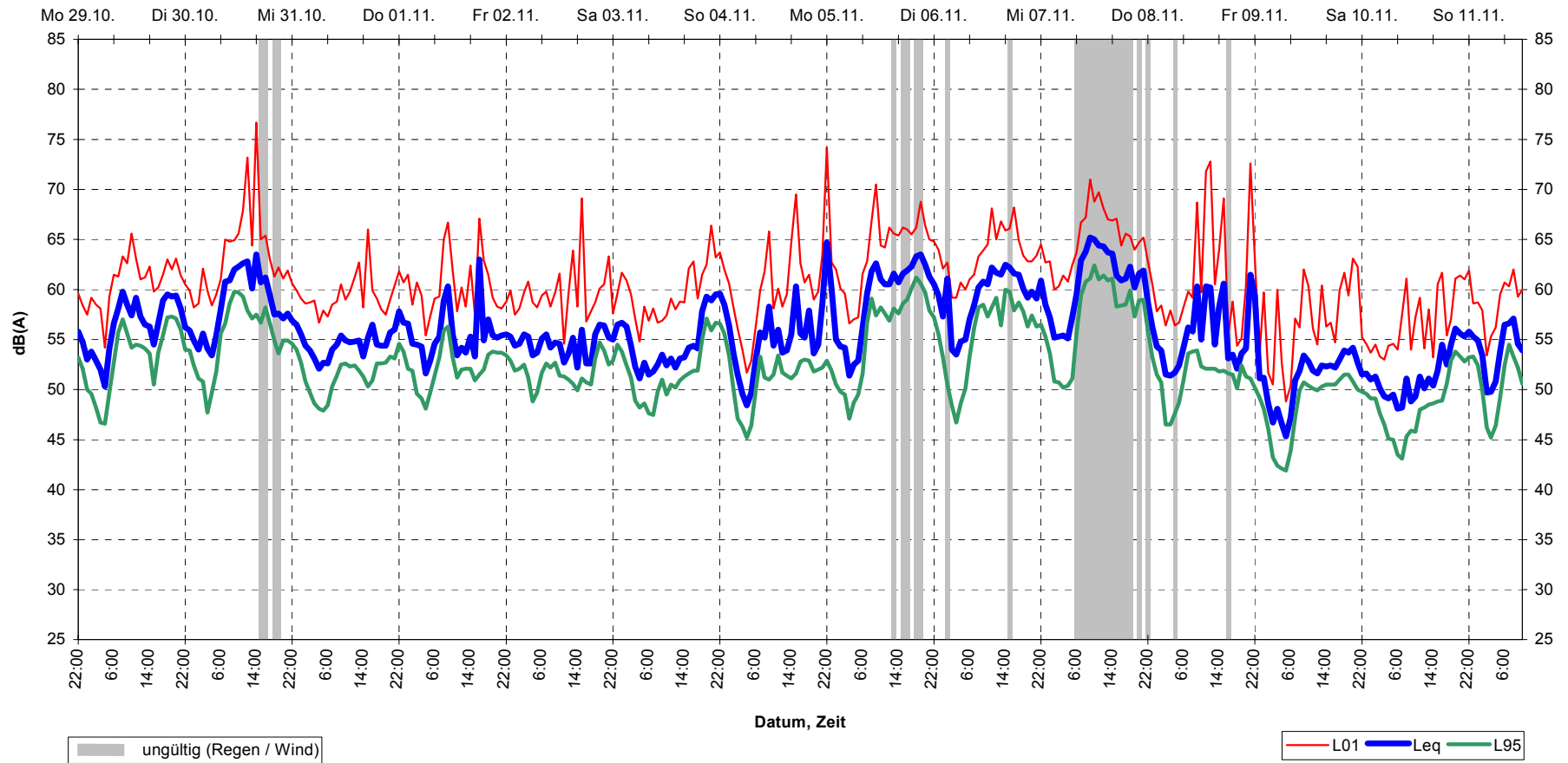
Schalldruckpegel (Stundenmittel) Stuttgart, MP58 29.10.01 bis 12.11.01
